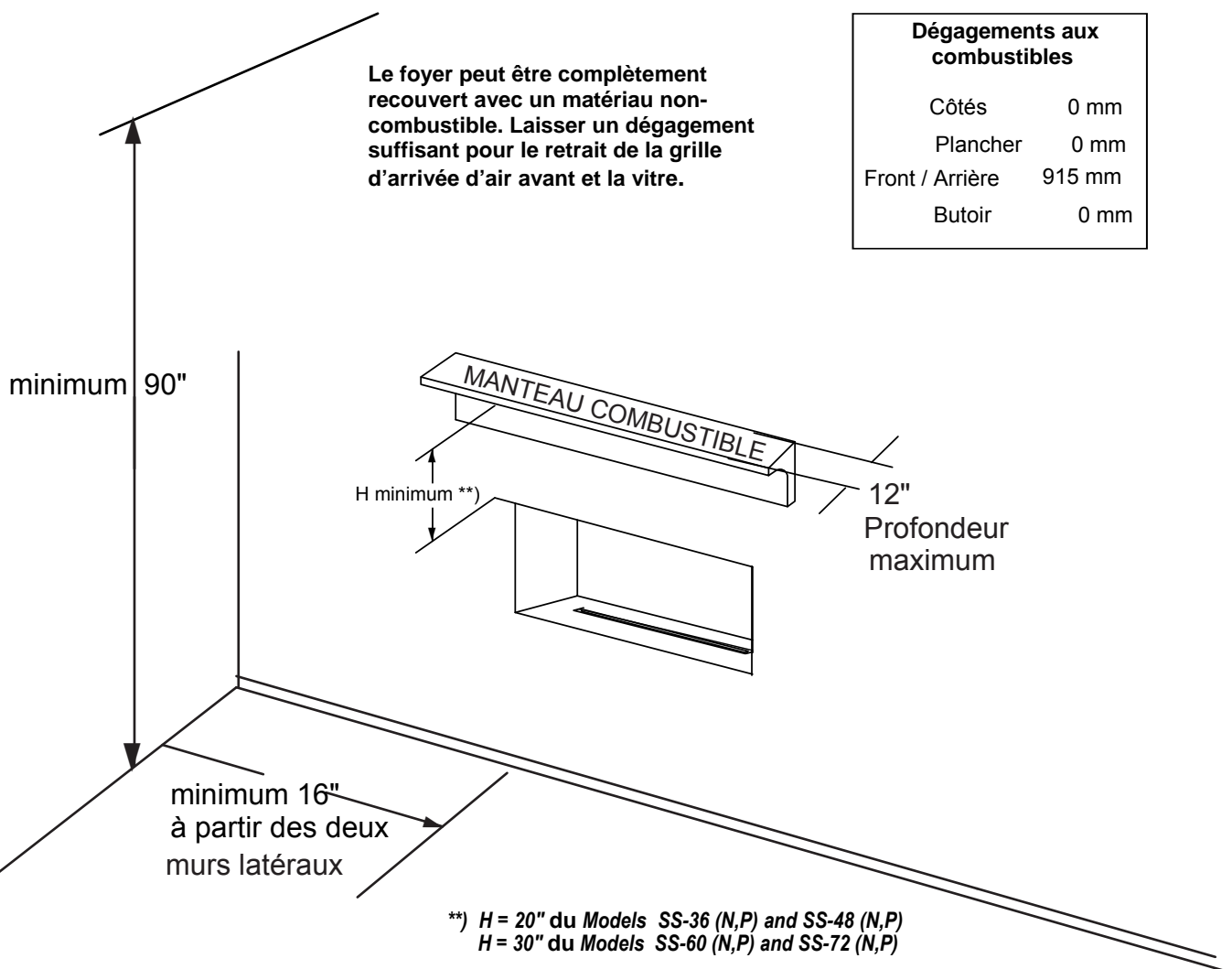
Schéma 6 - -Dégagements
